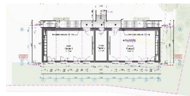
Grundriss EG
